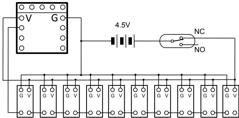
フルカラーシリアルLED連結基板(10個)
