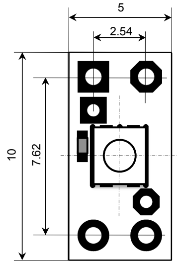
寸法図
